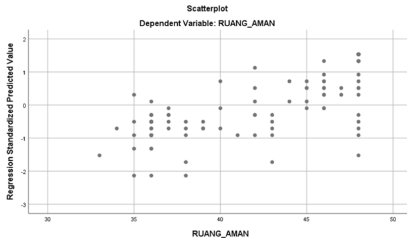
Gambar 2. Heteroskedastisitas
