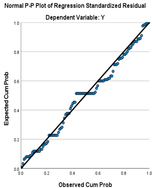
Gambar 1. Uji Normalitas
