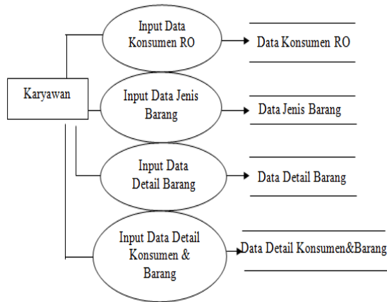
Gambar 3.5. DFD level 1
