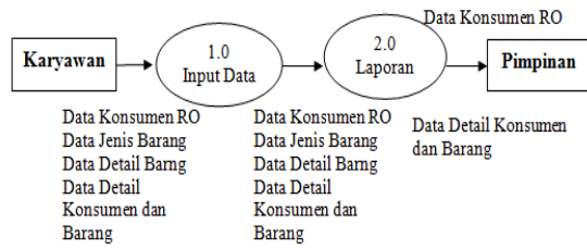
Gambar 3.4. DFD level 0
