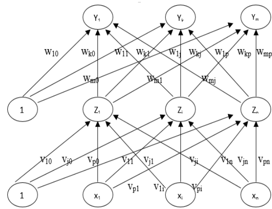
Gambar 6. Arsitektur Backpropagation
