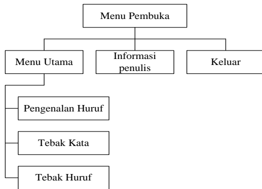
Gambar 3.2 Struktur Menu
