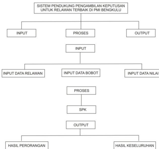
Gambar 9. Diagram HIPO
