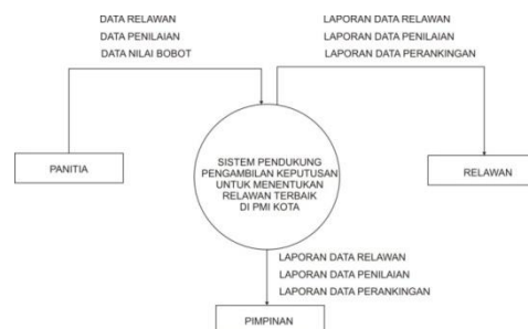
Gambar 5. Diagram Konteks
