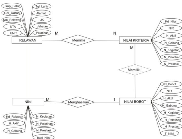
Gambar 10. ERD
