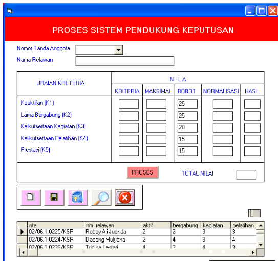
Gambar 17. Tampilan Menu Data Proses
