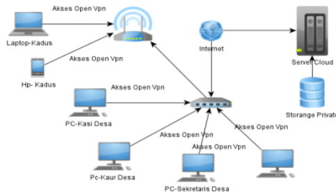
Gambar 3 Topologi jaringan ownCloud yang ditambah akses openVPN
