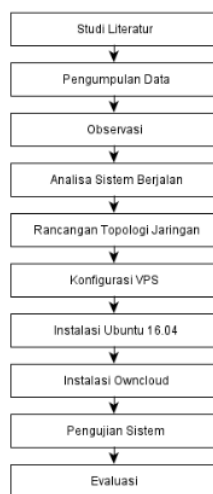
Gambar 1 Tahapan Penelitian
