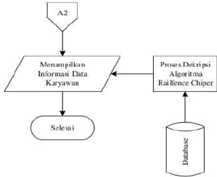
Gambar 6 Flowchart Informasi Data Karyawan
