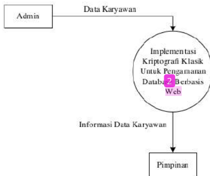
Gambar 7 Diagram Konteks
