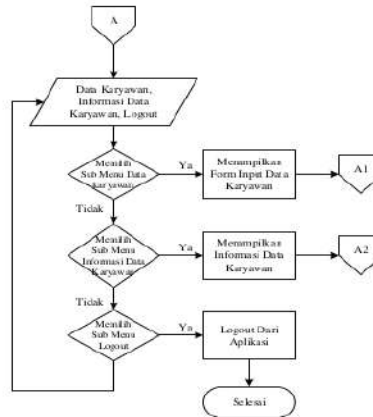
Gambar 4 flowchart menu utama
