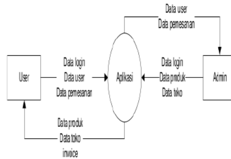
Gambar 4 DFD Diagram Konteks
