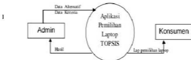
Gambar 3.2 Diagram Konteks
