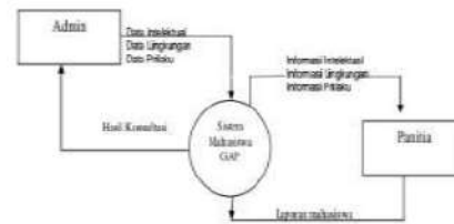
Gambar 3.2 Diagram Konteks
