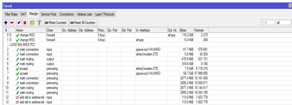
Gambar 4 Konfigurasi Load Balancing
