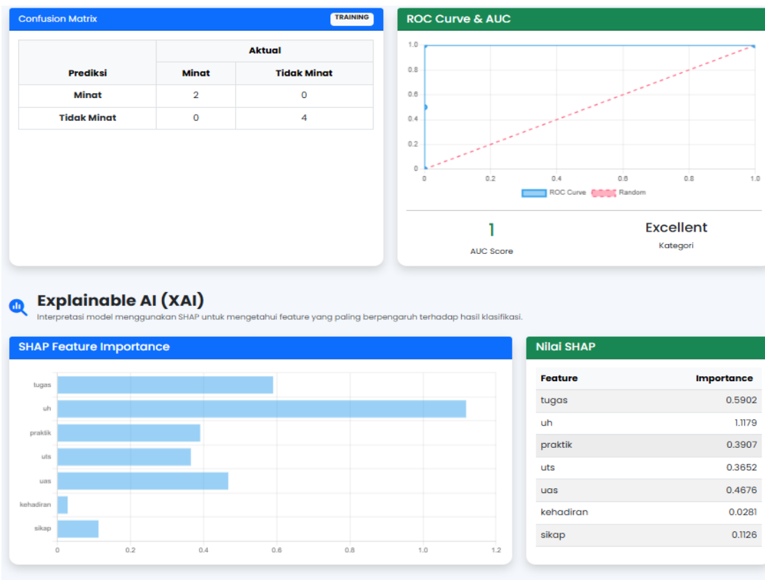
Gambar 3. Ringkasan evaluasi XGBoost dan interpretasi SHAP pada sistem penelitian
