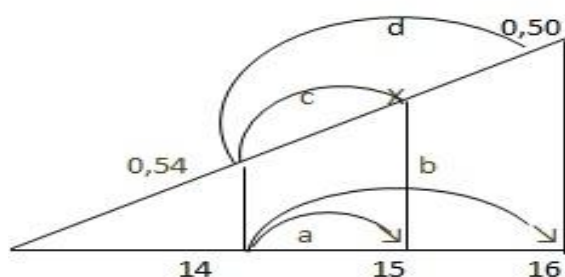
Gambar 3. Interpolasi n=15
