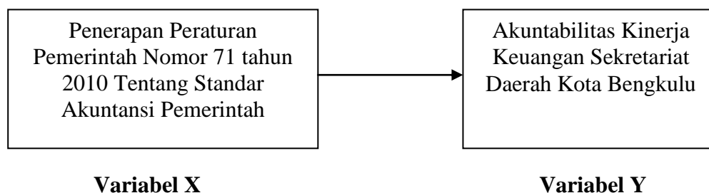
Gambar 1. Kerangka Analisis
