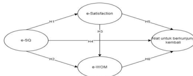
Gambar 1. Kerangka Berpikir
