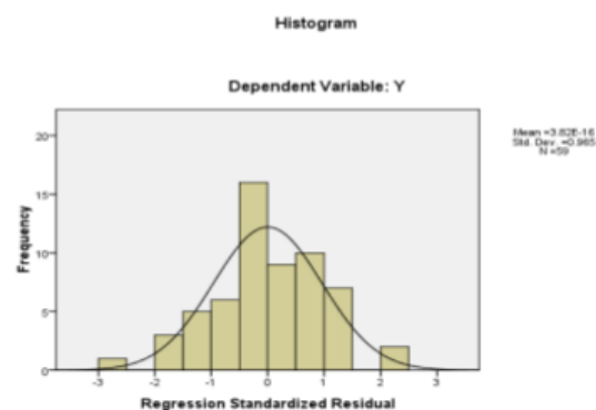
Gambar 2. Kurva Normal
