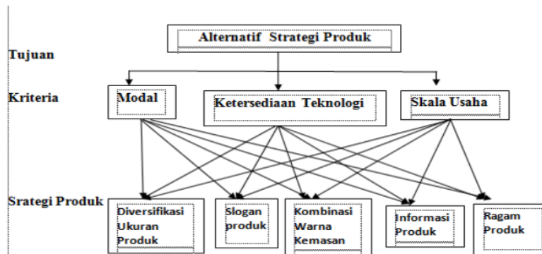
Gambar 8. Struktur Hirarki dalam AHP Pemilihan Alternatif Strategi Produk Kopi
